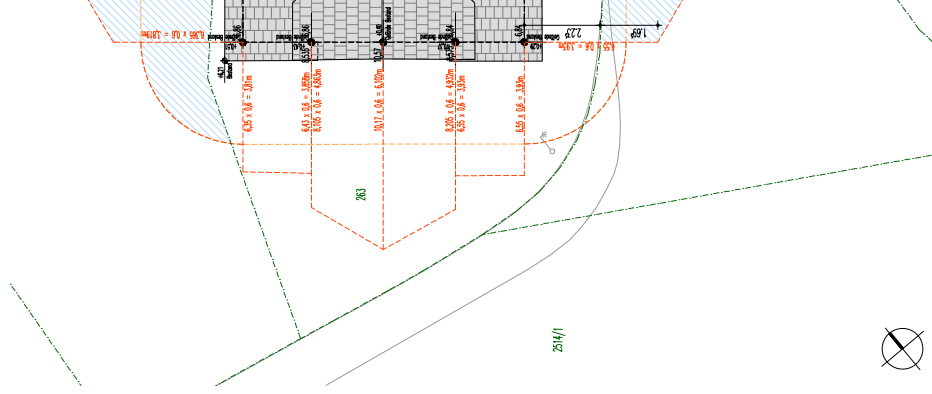
ABSTANDSFLÄCHENPLAN M 1:100
